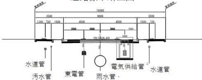
道路標準断面図
